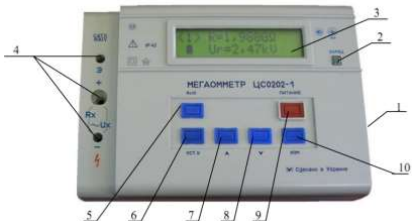
Рисунок 6 – Зовнішній вигляд мегомметра ЦС0202-1:
