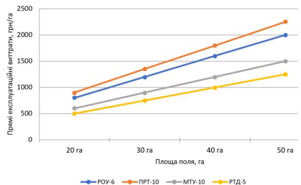
Рис. 6. Залежність ефективності використання мобільних машин для подрібнення та розкидання органічних добрив від прямих експлуатаційних витрат: 1 – МТУ-10, 2 – ПРТ-10, 3 – РОУ-6, 4 – РТД-5
