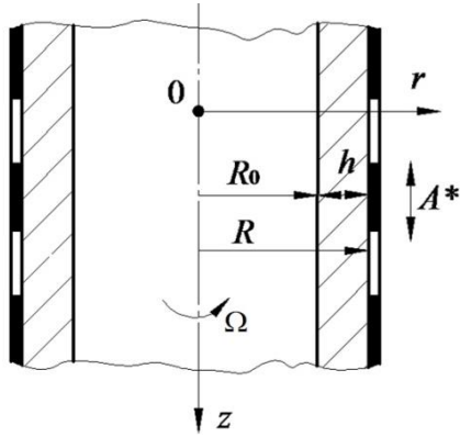
Рис. 1. Розрахункова схема
